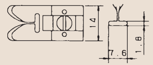
Presserfuß / Presser foot: 91-154 903-93
