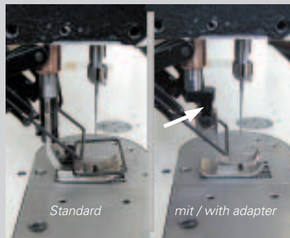
Nähfußadapter für Nähwerkzeuge der PFAFF 938 Sewing foot adapter for the parts set of the PFAFF 938
