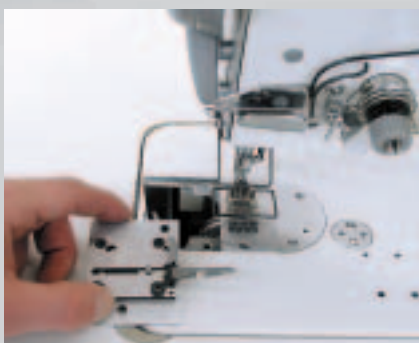
Zuverlässiger und sicherer Fadenabschneider -900/93 Extremely reliable thread trimming mechanism -900/93
