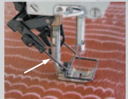
Fadenwischereinrichtung -909/93 für sauberen Nahtanfang Thread wiper mechanism -909/93 for clean seam start
