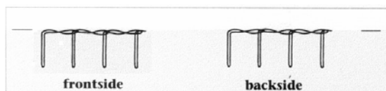
Edging stitch of ME – Serie 18
